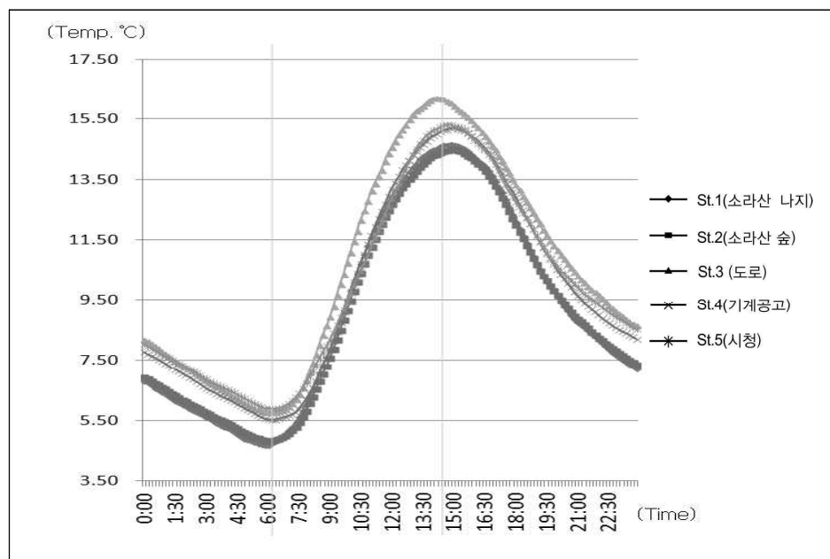
그림 4. 지점별 하루 동안의 평균 온도변화
