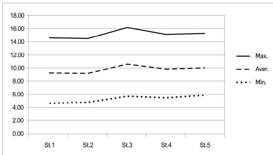
그림 3. 관측기간 내 지점별 하루 동안의 온도 비교
